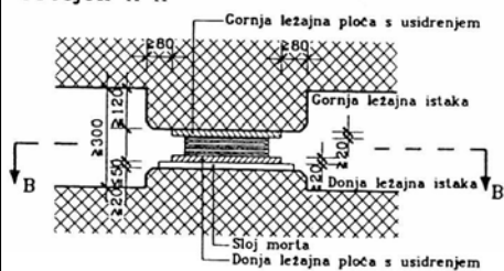
Presjek A-A
