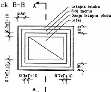
Presjek B-B
